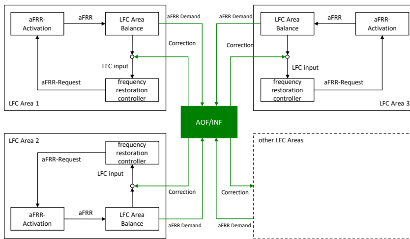
Obr. 2.7 Koncept riadenia Picasso a IGCC (IN)
