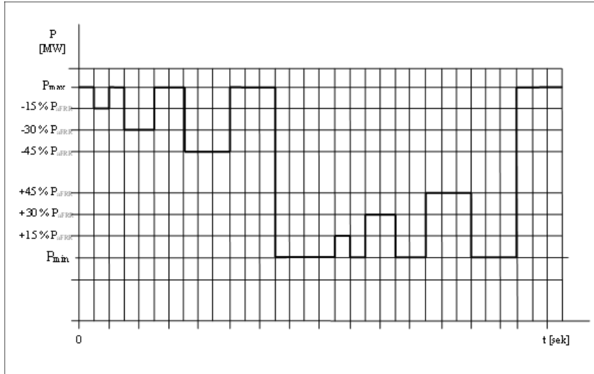
Obr. B5.2b Skúšobný signál pre overovanie aFRR+/aFRR-
