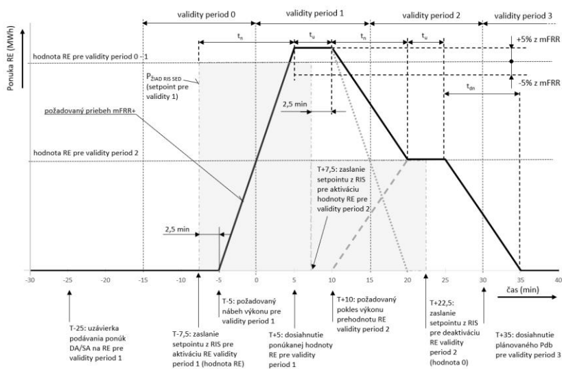
Obr.B2.20 Požadovaný priebeh výkonu pri certifikácii mFRR+ po aktivácii typu SA – zmena aktivovanej hodnoty RE platnej pre validity period 1 na hodnotu RE platnú pre validity period 2
