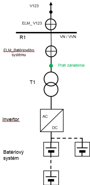
Obr. B1.11 Prah a svorky batériového systému.
