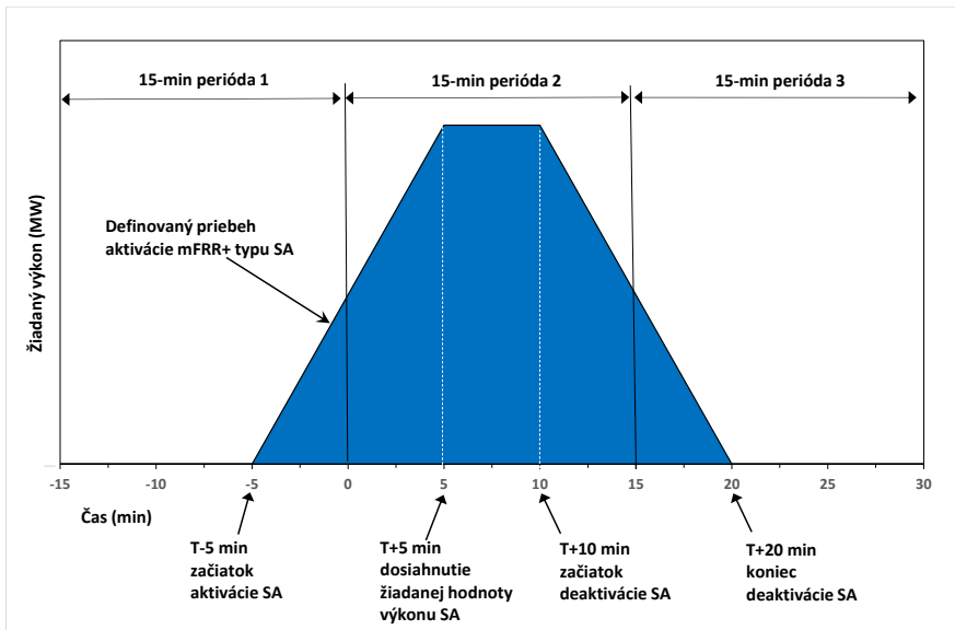
Obr. 4.3.2. a) Definovaný priebeh aktivácie typu SA.
