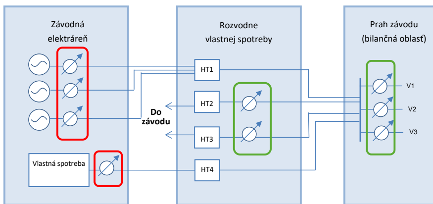
Obr. B1.8 Koncepcná schéma zapojenia závodnej elektrárne v rámci závodu
