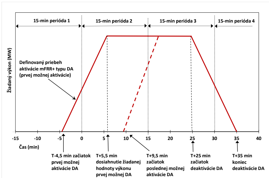
Obr. 4.3.2. b) Definovaný priebeh aktivácie typu DA.
