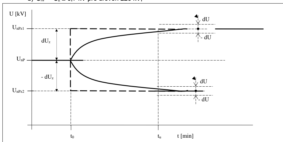
Obr. B2.1821 Požadovaný priebeh napätia v pilotnom uzle po skokovej zmene žiadanej hodnoty
