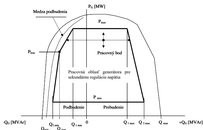
Obr. B2.4922 Obecný P-Q diagram generátora
