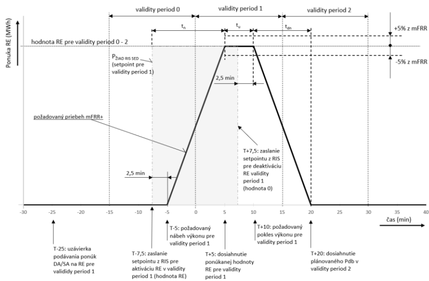
Obr. B2.18 Požadovaný priebeh výkonu pri certifikácii mFRR+ po aktivácii typu SA
