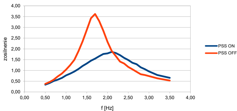
Obr. B5.5 Príklad amplitúdovej frekvenčnej charakteristiky činného výkonu SG
