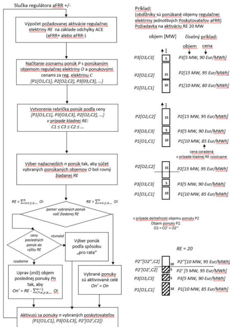
Obr. B2.5 Proces prerozdelenia žiadaneho výkonu v aFRR+/aFRR- (Merit order)
