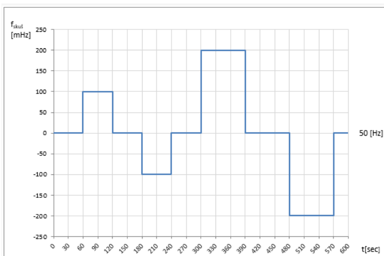
Obr. B5.1 Skúšobný signál pre overenie akcieschopnosti FCR
