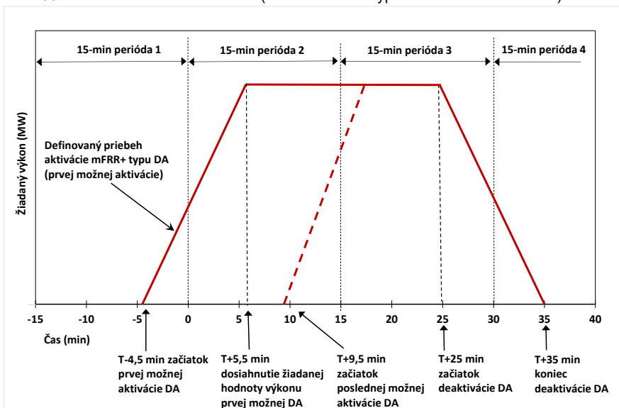
Obr. B4.2 Definovaný priebeh aktivácie typu DA
