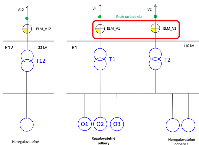
Obr. B1.9 Prah odberateľa
