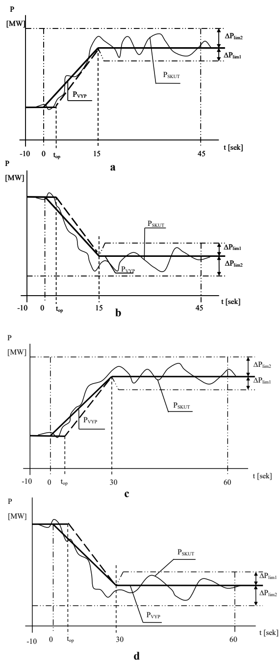
Obr. B2.3 Požadovaný priebeh výkonu pri certifikácii po aktivácii FCR
