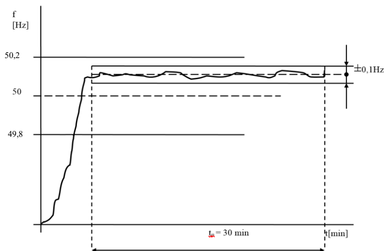
Obr. B5.4 Požadovaný priebeh frekvencie na určenej prípojnici pri "Štarte z tmy" pri ustálení
