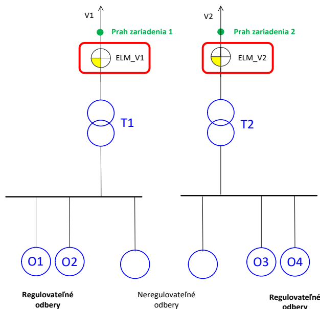
Obr. B1.10 Prah odberateľa s dvoma zariadeniami
