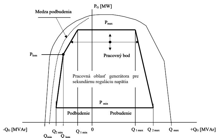
Obr. B2.15 Obecný P-Q diagram generátora
