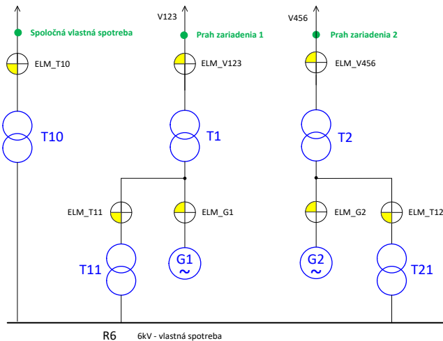
Obr. B1.5 Spoločné meranie vlastnej spotreby
