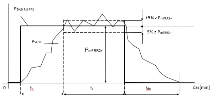
Obr.B2.9 Požadovaný priebeh výkonu pri certifikácii po aktivácii mFRR3+
