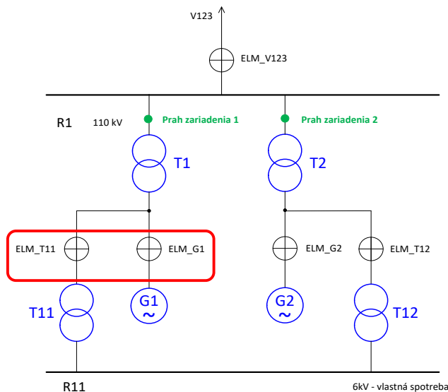
Obr. B1.4 Spoločné meranie
