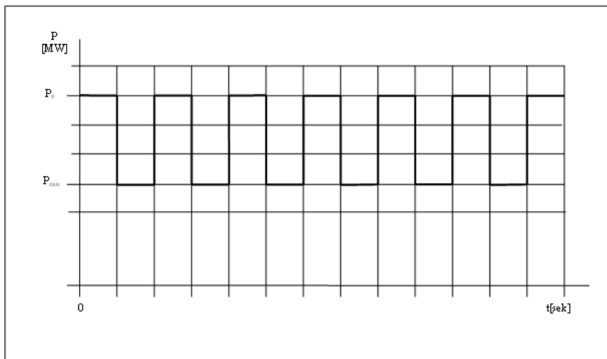
Obr. B5.2c Skúšobný signál pre overovanie aFRR+/aFRR-
