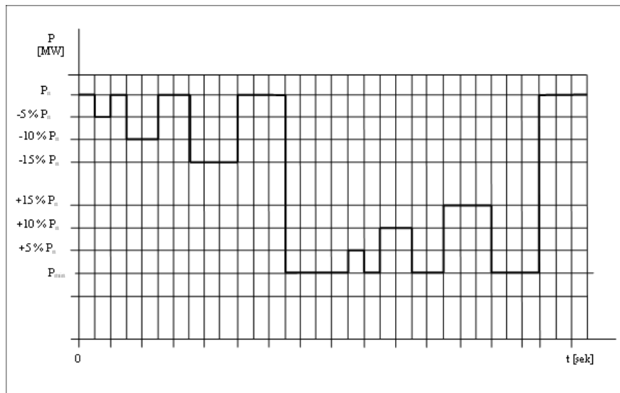
Obr. B5.2a Skúšobný signál pre overovanie aFRR+/aFRR-
