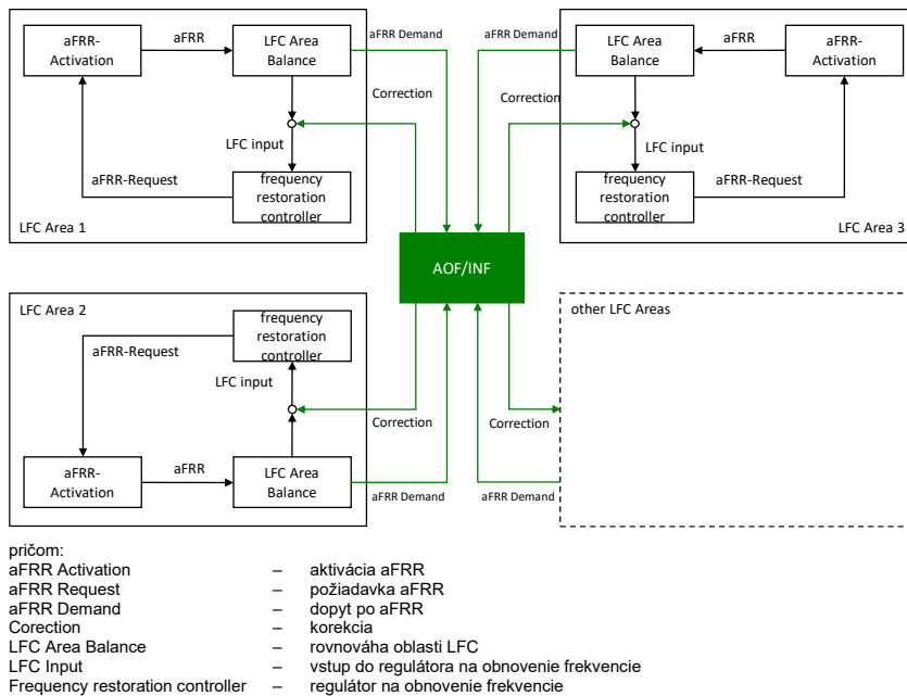
Obr. 2.7 Koncept riadenia Picasso a IGCC (IN)
