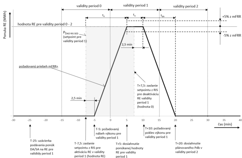
Obr. B2.11 Požadovaný priebeh výkonu pri certifikácii mFRR+ po aktivácii typu SA
