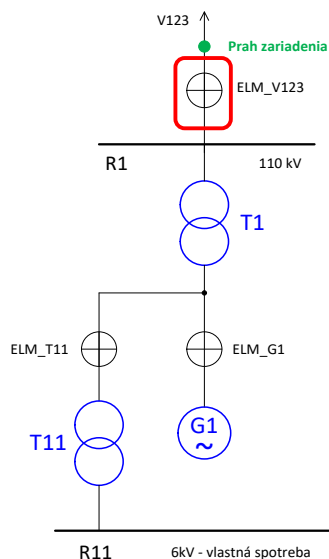
Obr. B1.2 Meranie za blokovým transformátorom
