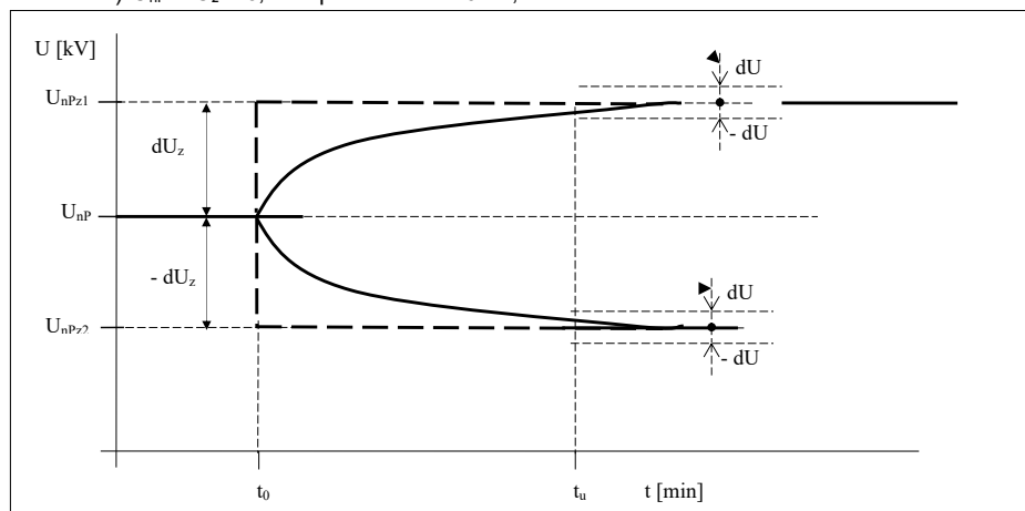
Obr. B2.14 Požadovaný priebeh napätia v pilotnom uzle po skokovej zmene žiadanej hodnoty
