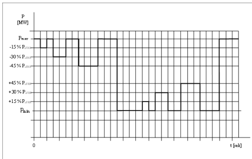
Obr. B5.2b Skúšobný signál pre overovanie aFRR+/aFRR-
