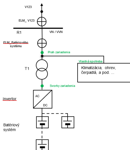
Obr. B1.11 Prah a svorky batériového systému.
