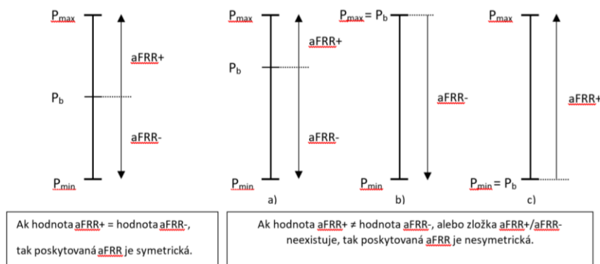
Obr.B2.8 Rozlíšenie typu aFRR.
