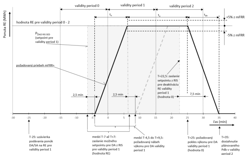
Obr.B2.12 Požadovaný priebeh výkonu pri certifikácii mFRR+ po aktivácii typu DA
