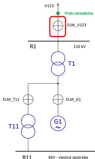
Obr. B1.2 Meranie za blokovým transformátorom
