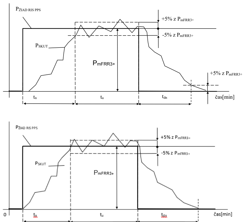
Obr.B2.9 Požadovaný priebeh výkonu pri certifikácii po aktivácii mFRR3+
