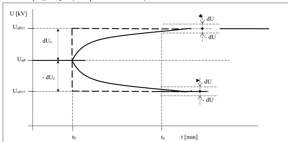
Obr. B2.14 Požadovaný priebeh napätia v pilotnom uzle po skokovej zmene žiadaneho napätia
