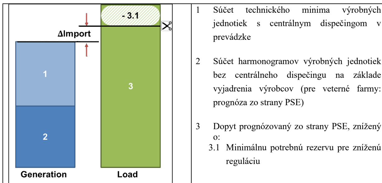
Obr. 2: Určenie externých obmedzení v smere dovozu (rezerva vo výrobných kapacitách dostupných pre potenciálne dovozy) v rámci výpočtu kapacity pre denný trh.
