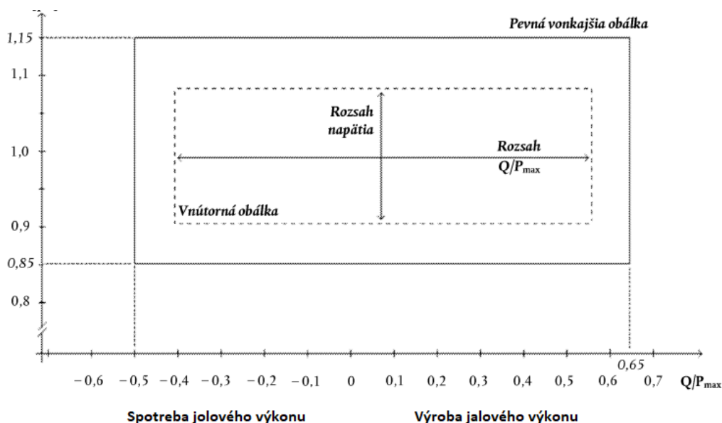
Závislosť U-Q/P_{\max} pre jednotky parku zdrojov jednosmerne pripojené do PS
